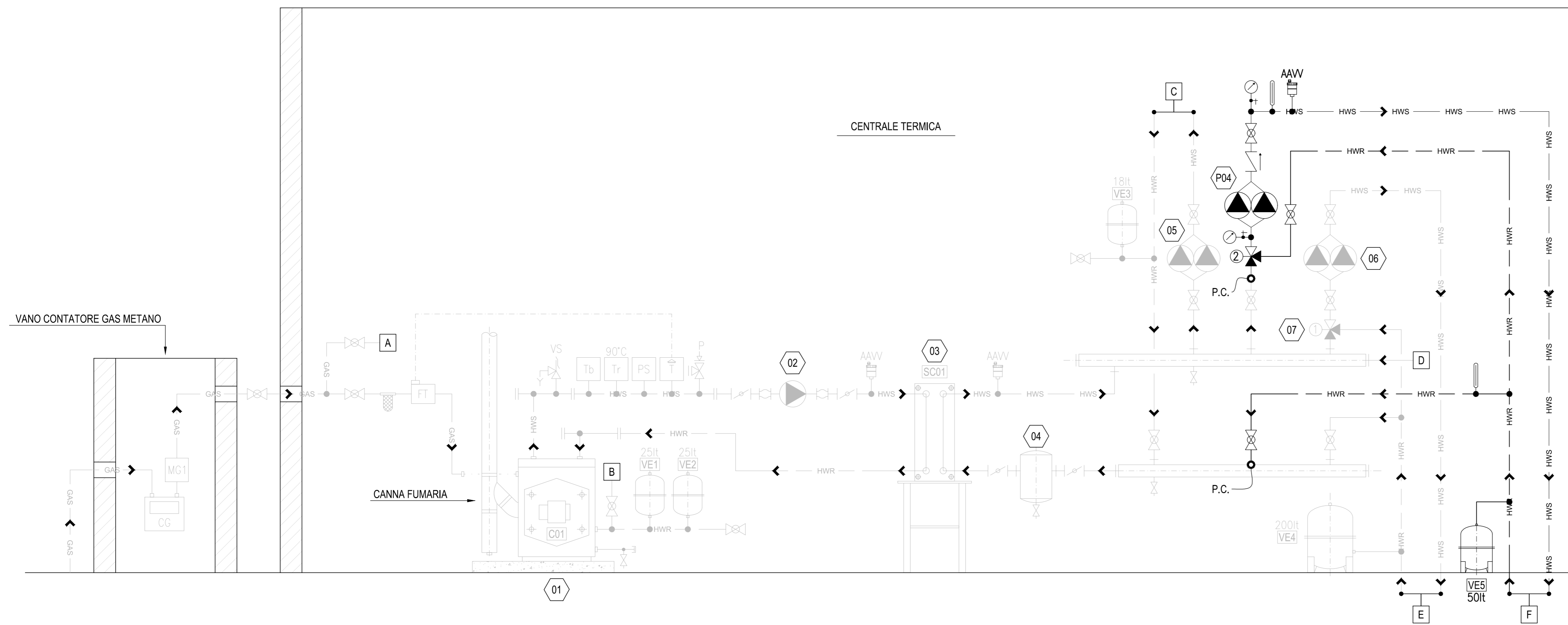
SCHEMA FUNZIONALE RISCALDAMENTO NUOVO NO SCALA
