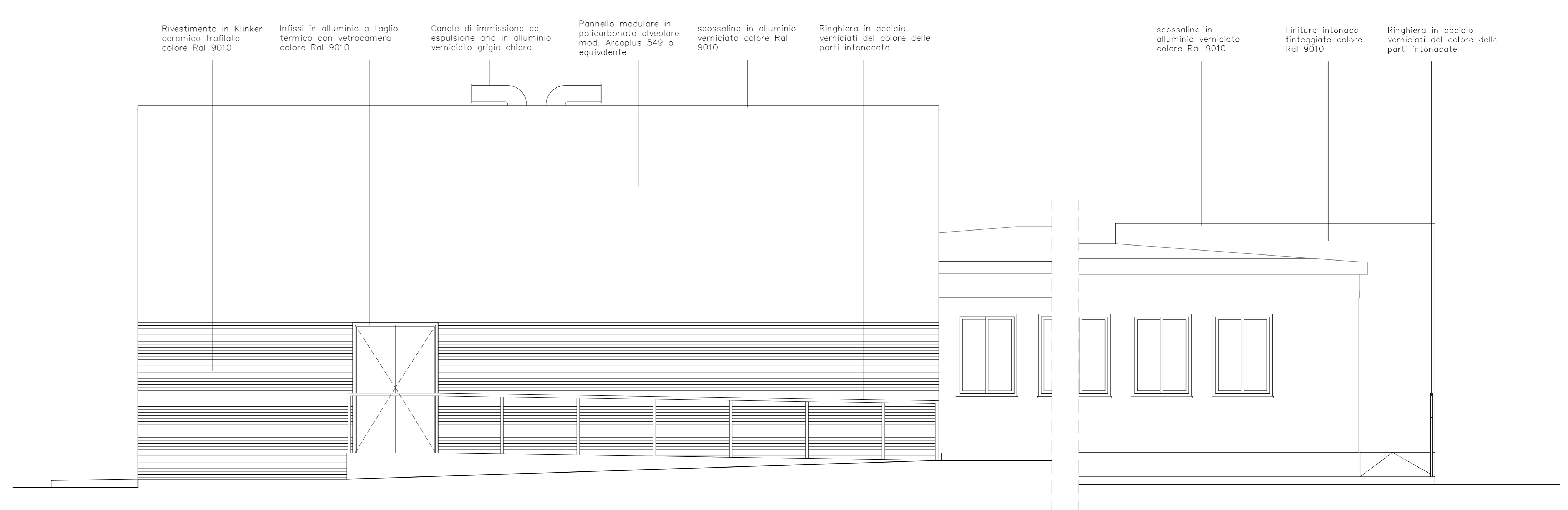
Prospetto Nord
