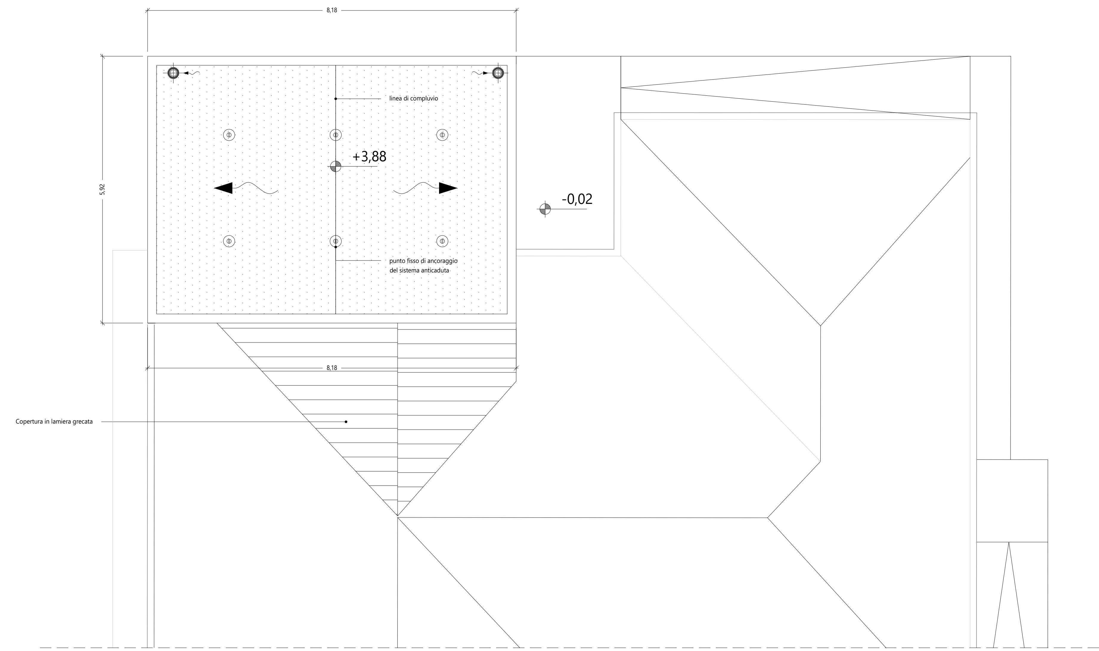
PIANTA PIANO TERRA - Blocco Ovest (Servizi Igienici)
