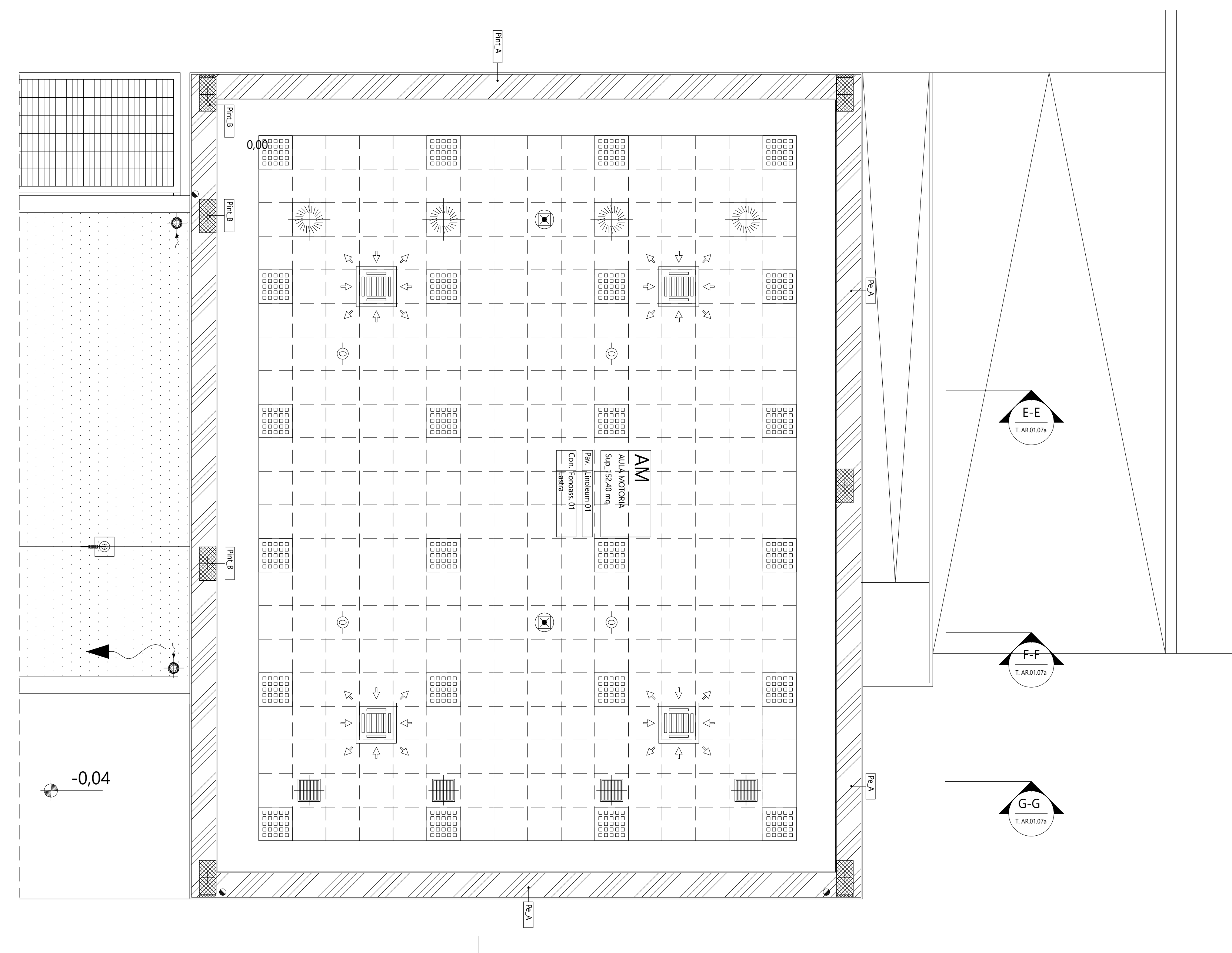
PIANTA QUOTA +3.95 - Blocco Est (Aula Motoria)
