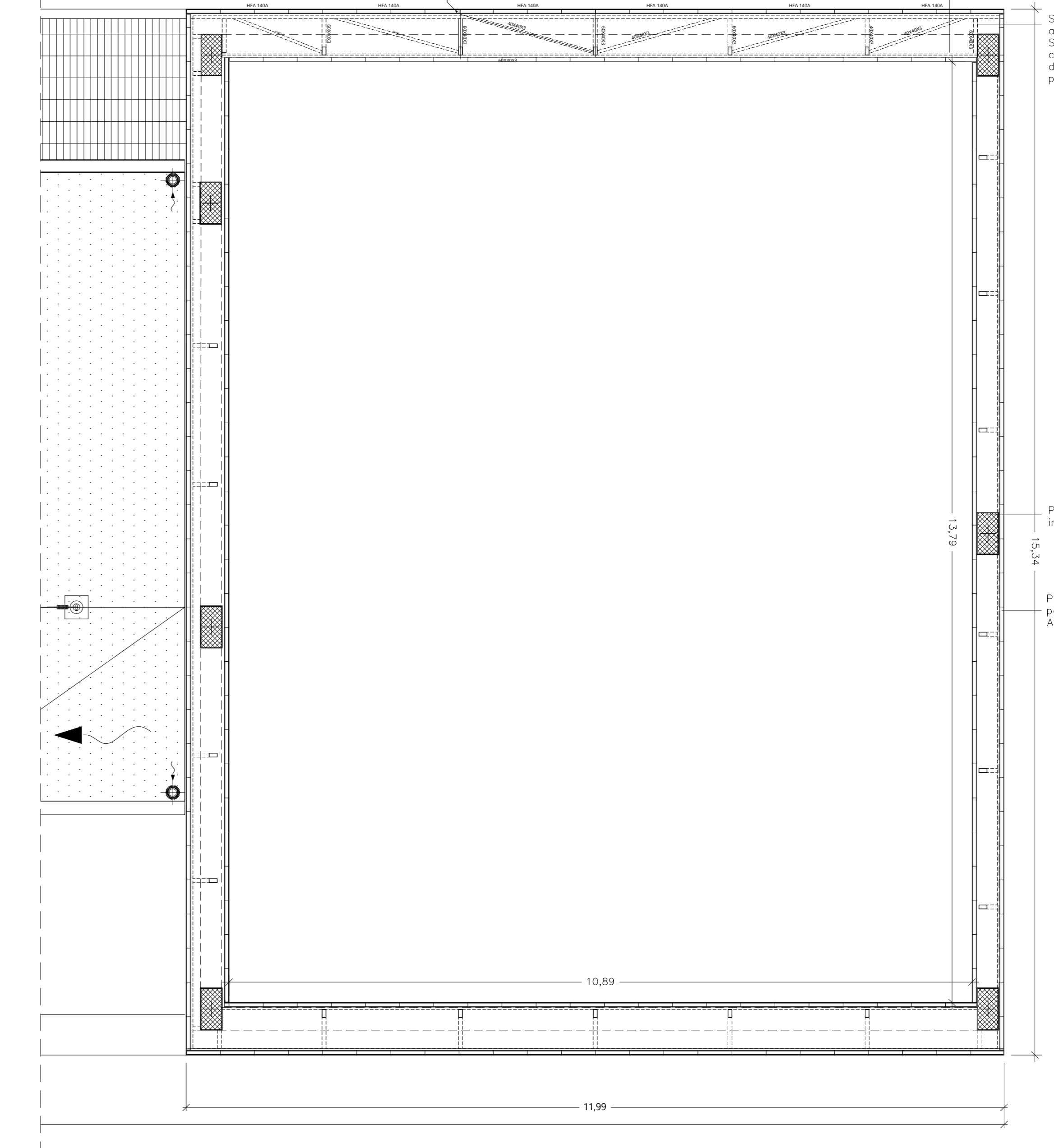
PIANTA QT 4,5 mt - Aula Motoria
