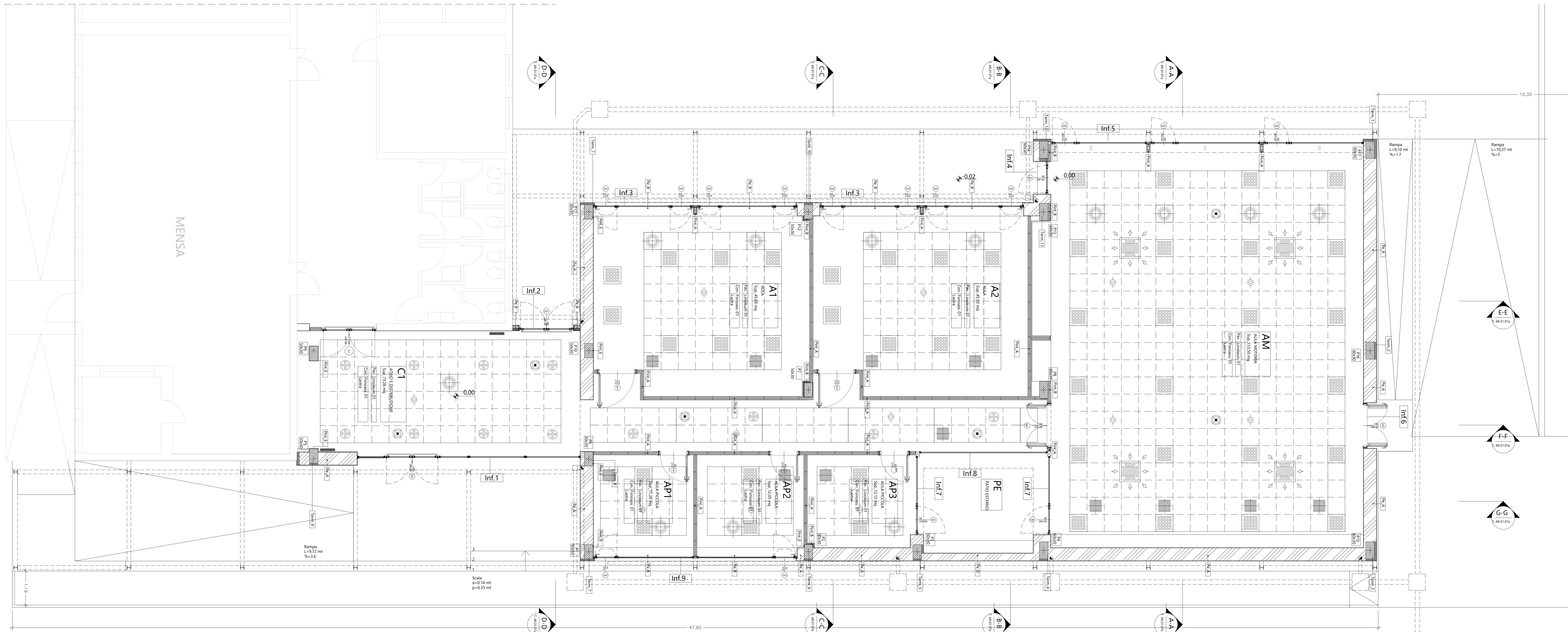
PIANTA PIANO TERRA - Blocco Est (Aule)
