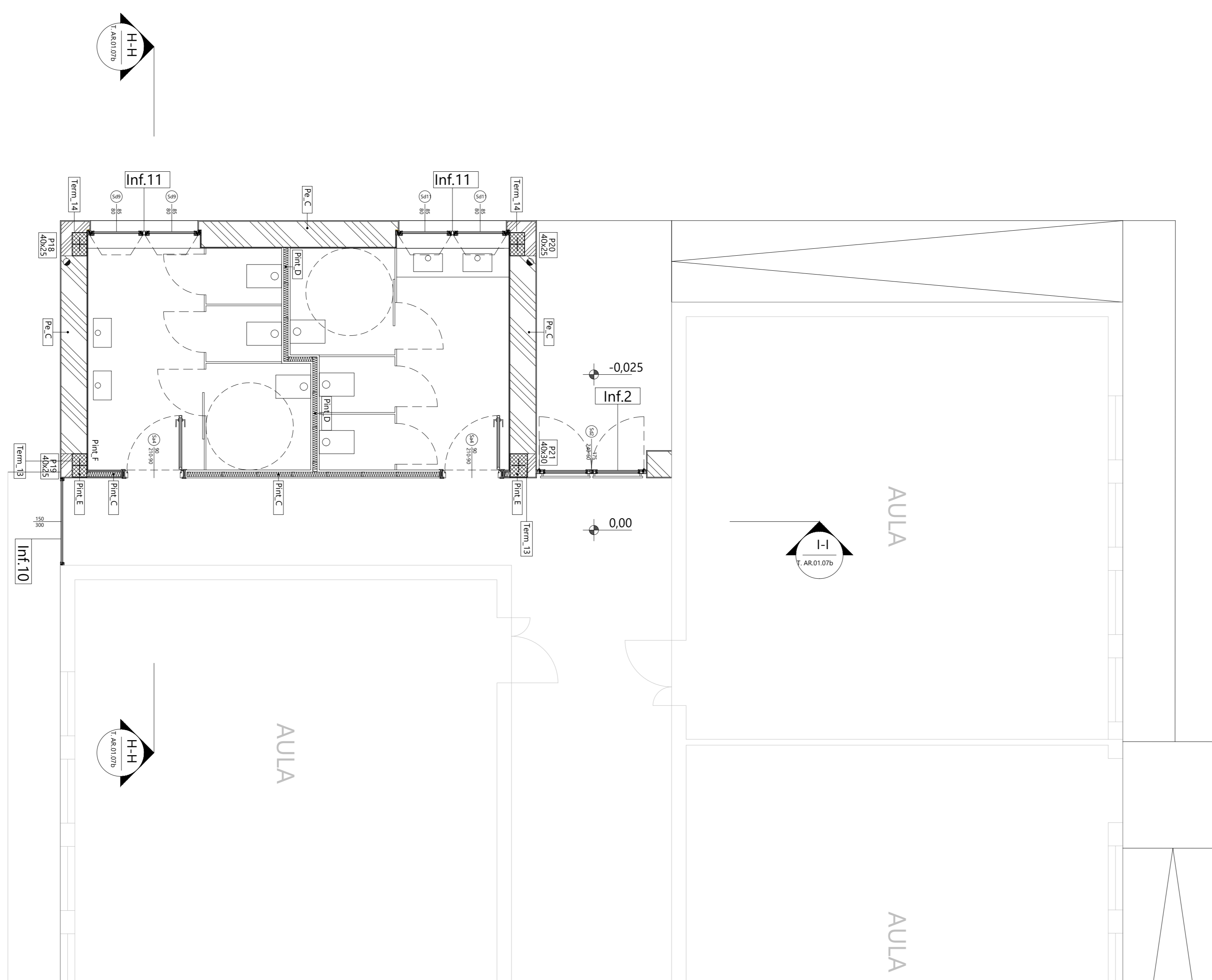
PIANTA PIANO TERRA - Blocco Ovest (Servizi Igienici)
